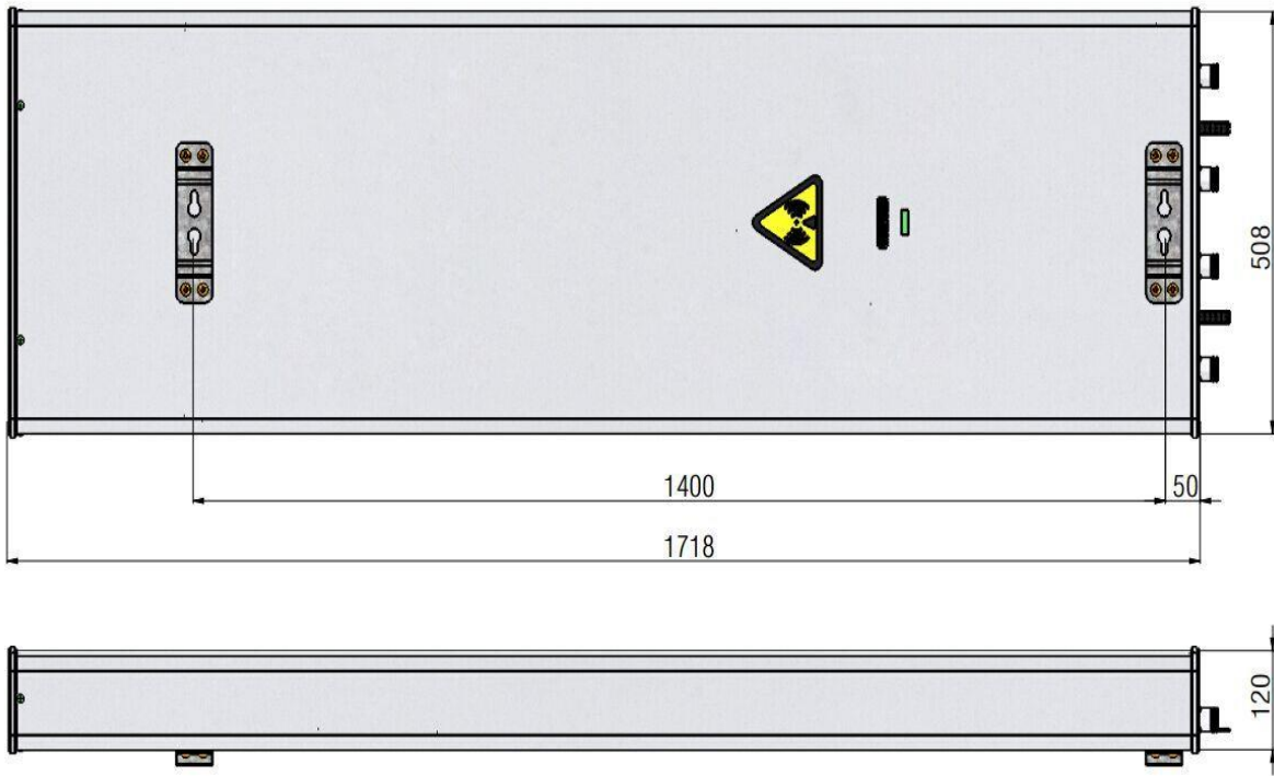
产品尺寸细节图
