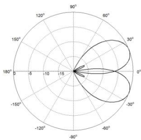
水平方向图
