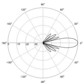
垂直方向图
